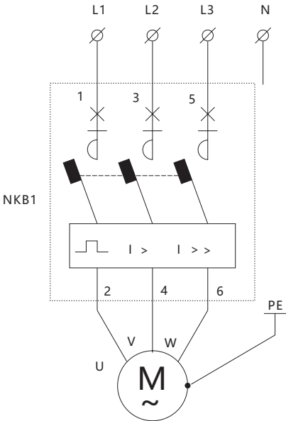
Рис. 6. Схема управления двигателем
