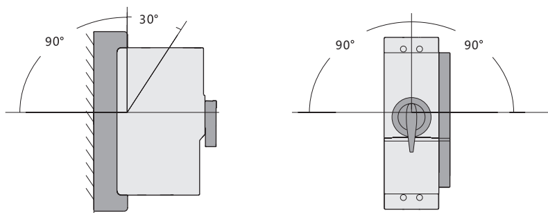
Рис. 9. Монтажные положения
